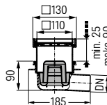
Rys.: Nr art. 40150.66
