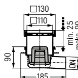
Rys.: Nr art. 40150.65
