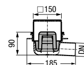
Rys.: Nr art. 40150.11
