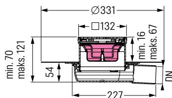
Rys.: Nr art. 44740.63M, 44750.63M
