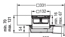
z systemem Lock&Lift i syfonem Megastop
